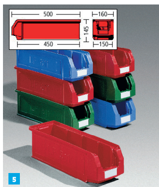
5 LF511: peso: 0.82 kg - capacità: 7.6 l - dim: 150x145x500 mm
