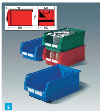
3 LF532: peso: 1.53 kg - capacità: 23.5 l - dim: 300x200x500 mm
