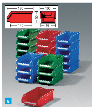
6 LF510: peso: 0.08 kg - capacità: 0.6 l - dim: 95x50x170 mm
