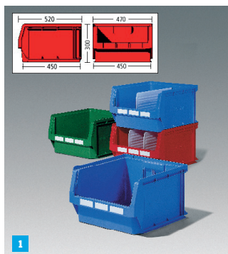
1 LF543: peso: 2.73 Kg - capacità: 57 l - Dim: 450x300x520 mm
